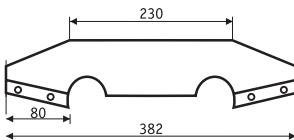
Снігозатримувач (півмісяць)
