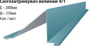
Снігозатримувач великий 4/1
